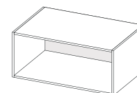
антресоль на шкаф 2-ств. высокий 900x400x570
