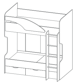
кровать - 5 1942x1700x992
