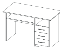
стол письменный 1100x750x600
