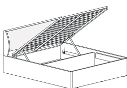
кровать арт. 033-М1 с ПМ* 1442/1642x935x2164
