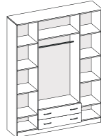
шкаф 4-ств. ящ. 1600x2016x525
