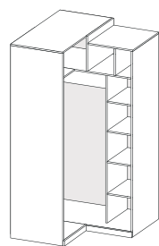
шкаф угловой ШкУ-1 954x2220x954
