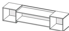
полка навесная 1,9 1940x450x260
