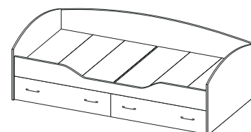
кровать 1942x700x860
