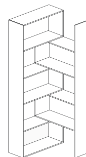
702X1860X702 (угловой вариант)
