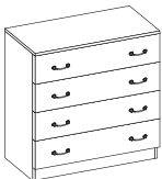
комод 964x830x450
