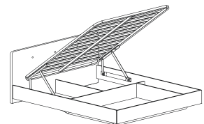
кровать арт. 031-М1 «Пуговицы» МЩ* с ЛДСП настилом/ с ПМ* 1545/1745x1000x2060
