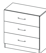
комод 750x750x390
