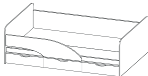
кровать - 3 лев./прав. 1942x700x862
