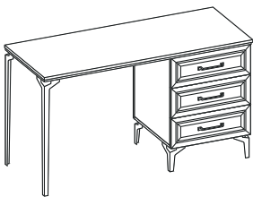
стол Ст-1 1310x755x500
