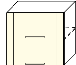
ШКАФ НАСТЕННЫЙ ДВУХДВЕРНЫЙ (с газлифтами)
