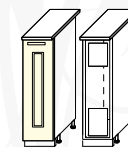
ШКАФ-СТОЛ С БУТЫЛОЧНИЦЕЙ
