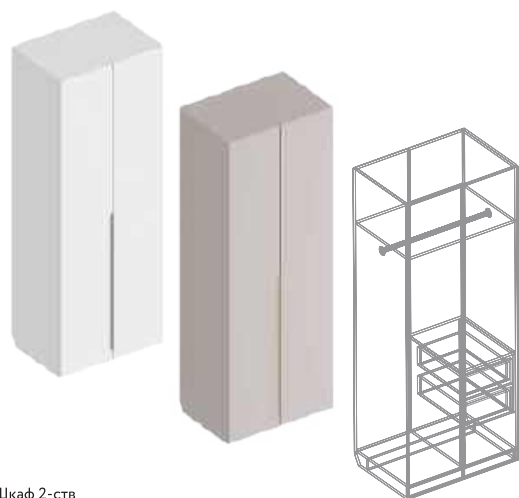
Шкаф 2-ств 800x550x2200
