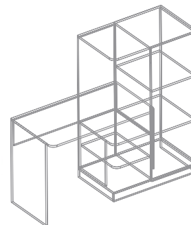
Стол письменный с пеналом ПРАВЫЙ (ориентир по пеналу) 1450x570x1280
