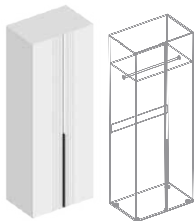
Шкаф 2-ств для одежды 800x520x2200
