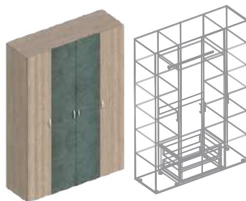
Шкаф 4-ств для одежды 1600x520x2300
