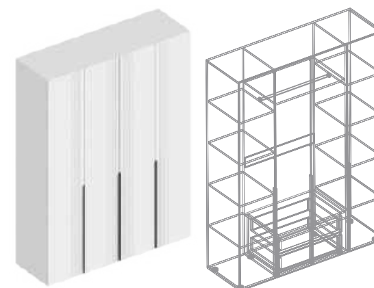
Шкаф 4-ств для одежды 1600x520x2200
