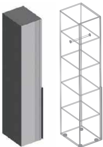
Пенал 1-ств с полками (штанга в комплекте) 400x520x2200
