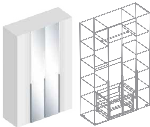
Шкаф 4-ств с зеркалом 1400x520x2200
