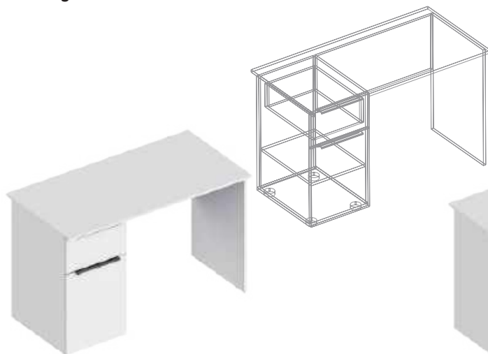
Стол письменный ЛЕВЫЙ (ориентир по тумбе) 1200x600x760
