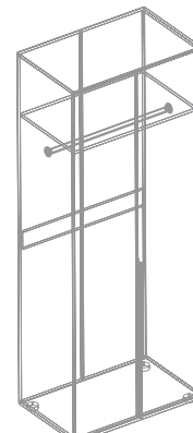
Шкаф 2-ств для одежды 800x500x2100
