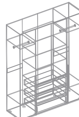
Шкаф 4-ств с 3 ящиками 1600x500x2100
