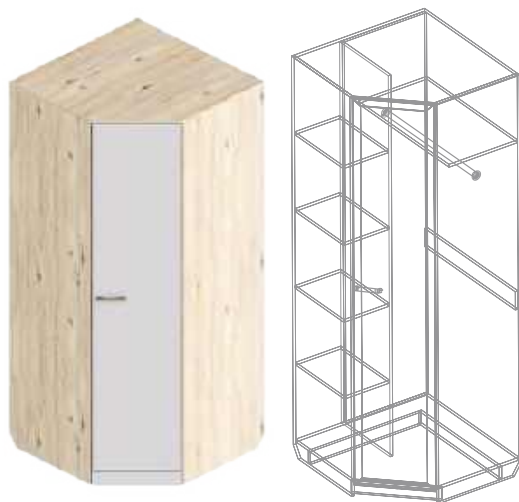
Шкаф угловой 940х940х2200
