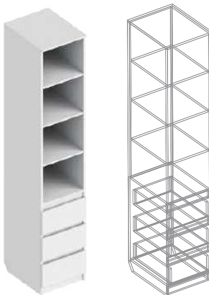
Пенал с 3 ящиками 400x500x2100
