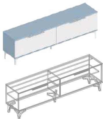
Тумба ТВ° 1600x350x350 °Можно использовать как навесную
