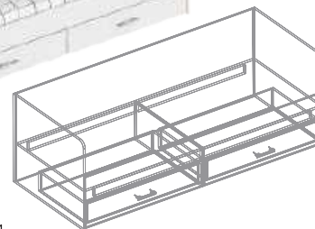
Кровать с 2 ящиками (основание ЛДСП) 832x2032x700 матрас 0,8x2,0
