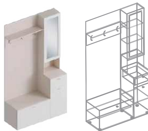
Прихожая Компакт ПРАВЫЙ (ориентир по зеркалу) 1200x450x2200
