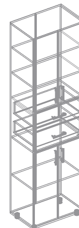
Шкаф с 2 ящиками (по центру) 600x390x2145
