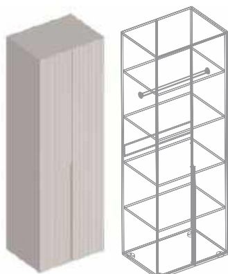
Шкаф 2-ств с полками (штанга в комплекте) 700x520x2200
