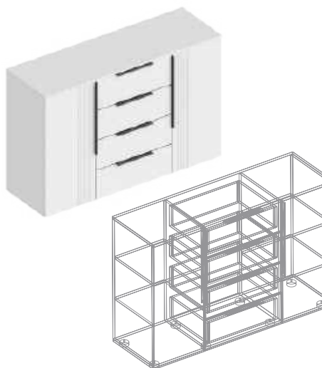
Комод 2-ств с 4 ящиками 1400x460x930
