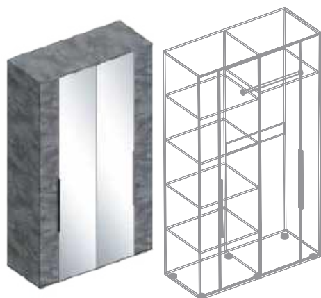
Шкаф 4-ств с зеркалом 1200x500x2100
