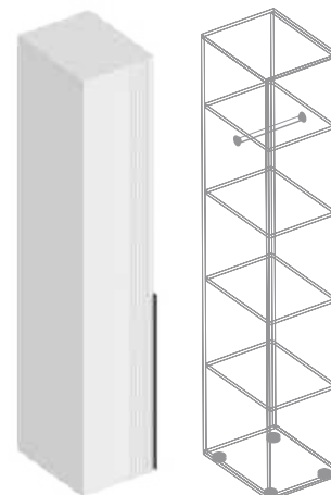
Пенал 1-ств с полками (штанга в комплекте) 400x520x2200
