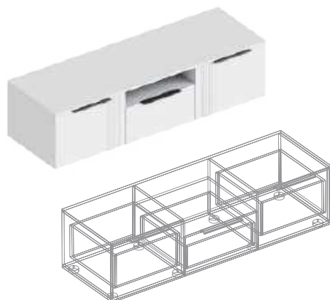
Тумба ТВ 1600x530x420
