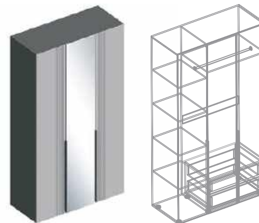
Шкаф 3-ств с зеркалом 1200x520x2200
