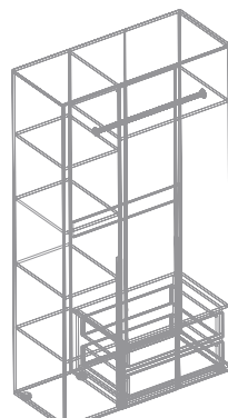
Шкаф 2-ств для одежды 800x520x2200
